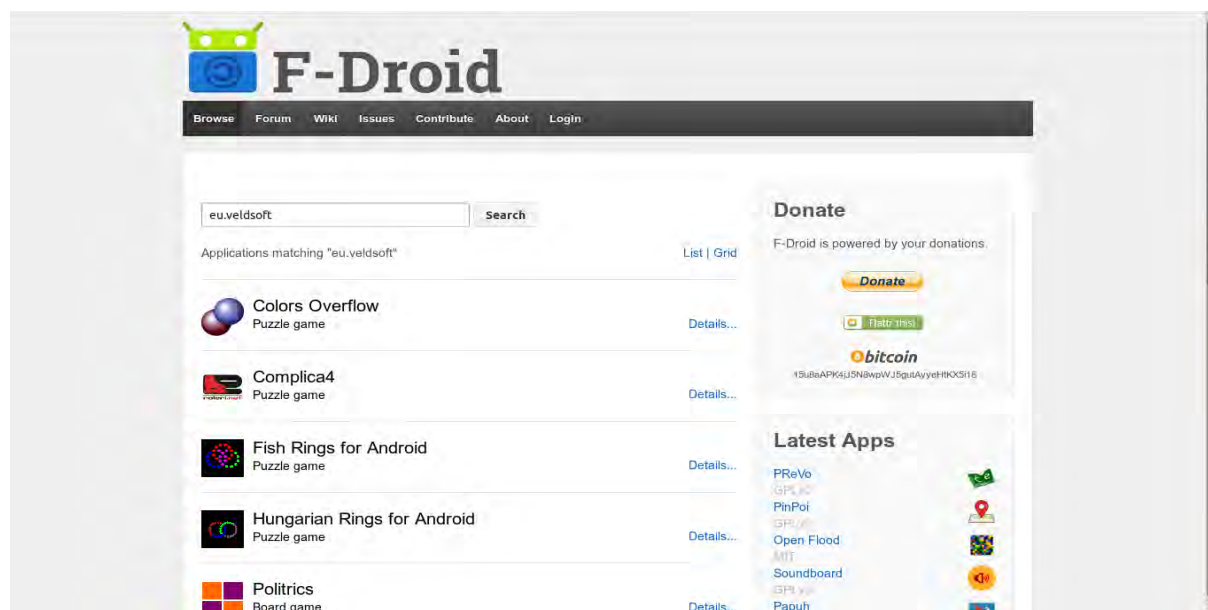
Фиг. 129 F-Droid.
