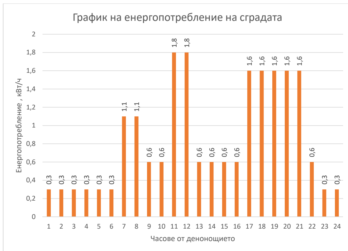
Фигура 4.2. График на енергопотребление на сграда \Sigma \text{Нел.} = 20,6 \text{ kW/h}
